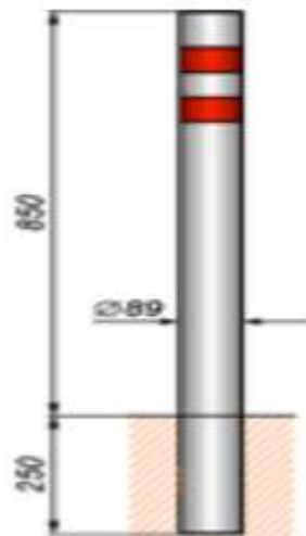
Рис. 4. Внешний вид и размеры столбика заграждения
